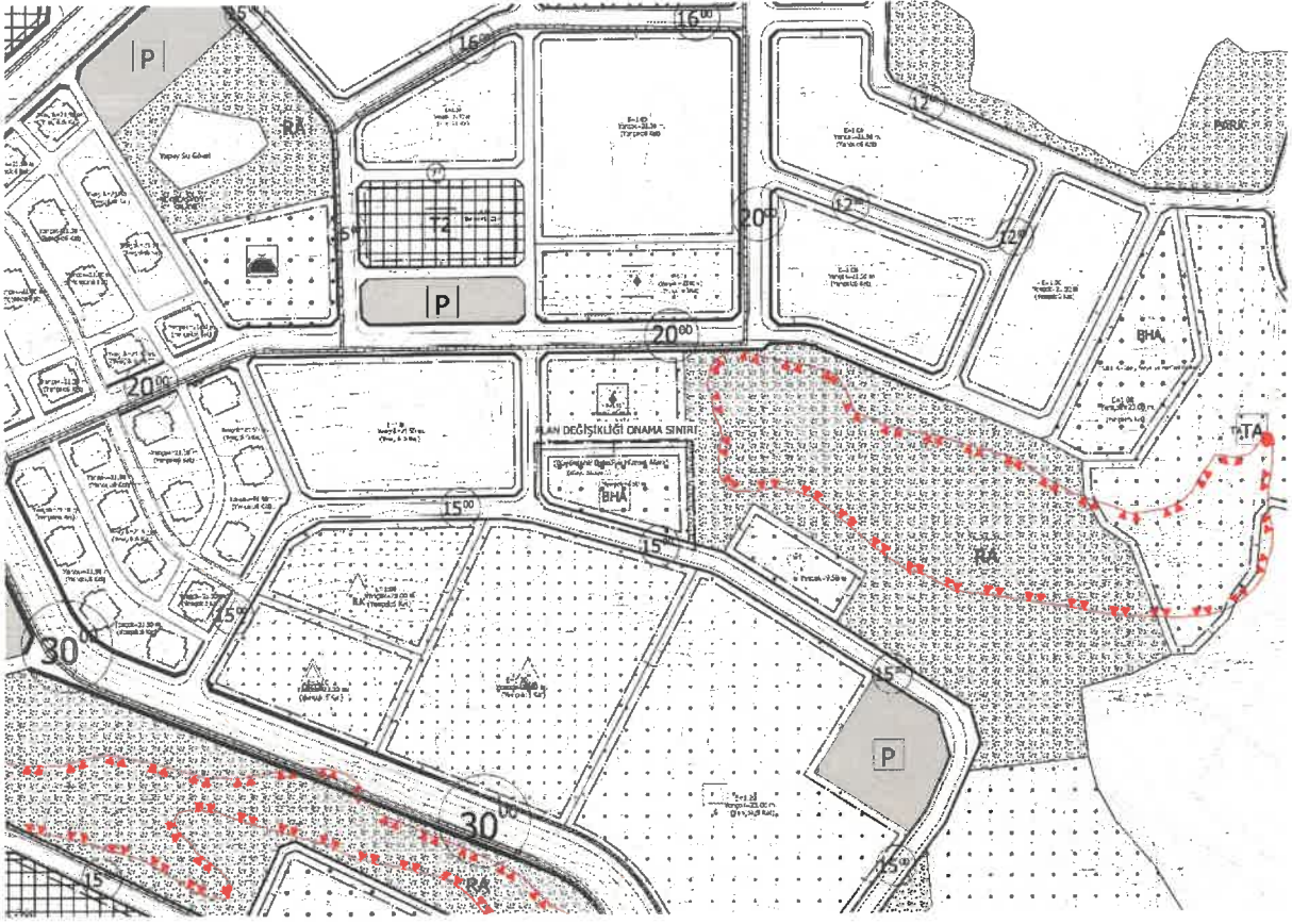
Şekil 9: Şehitkâmil İlçesi, Yalangöz Mahallesi Planlama Alanı Öneri 1/1000 Ölçekli Nazım İmar Planı
