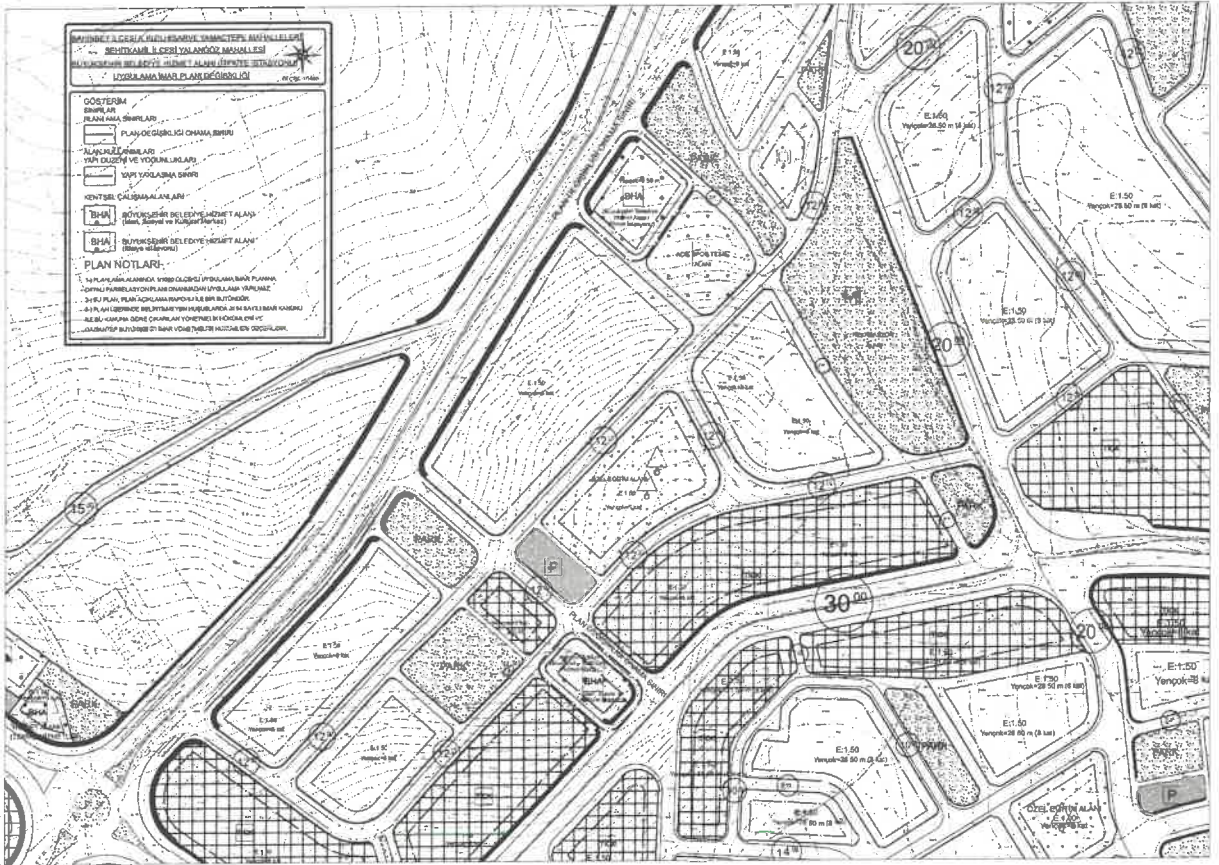
Şekil 8: Şahinbey İlçesi K.Kızılhisar Mahallesi Planlama Alanı Öneri 1/1000 Ölçekli Nazım İmar Planı
