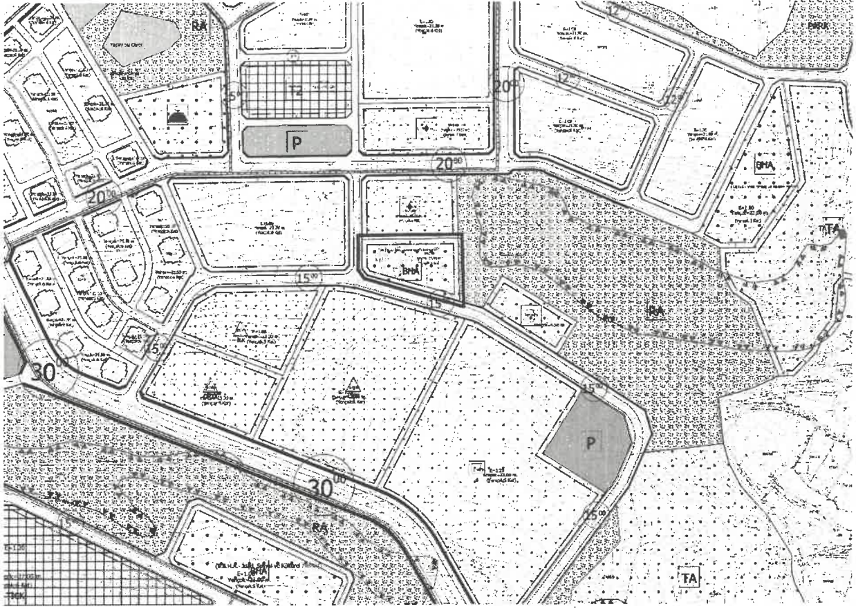
Şekil 6: Şehitkamil İlçesi, Yalangöz Mahallesi Planlama Alanı Mevcut 1/1000 Ölçekli Nazım İmar Planı
