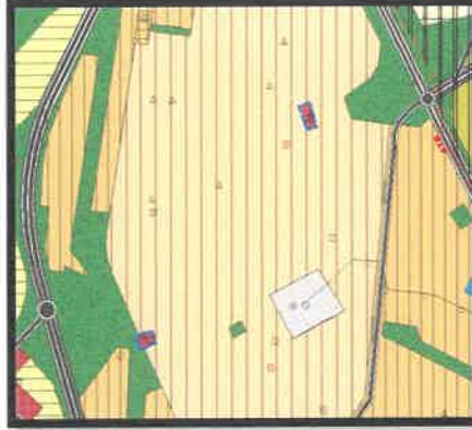
1/25.000 Ölçekli Öneri Nazım İmar Planı
