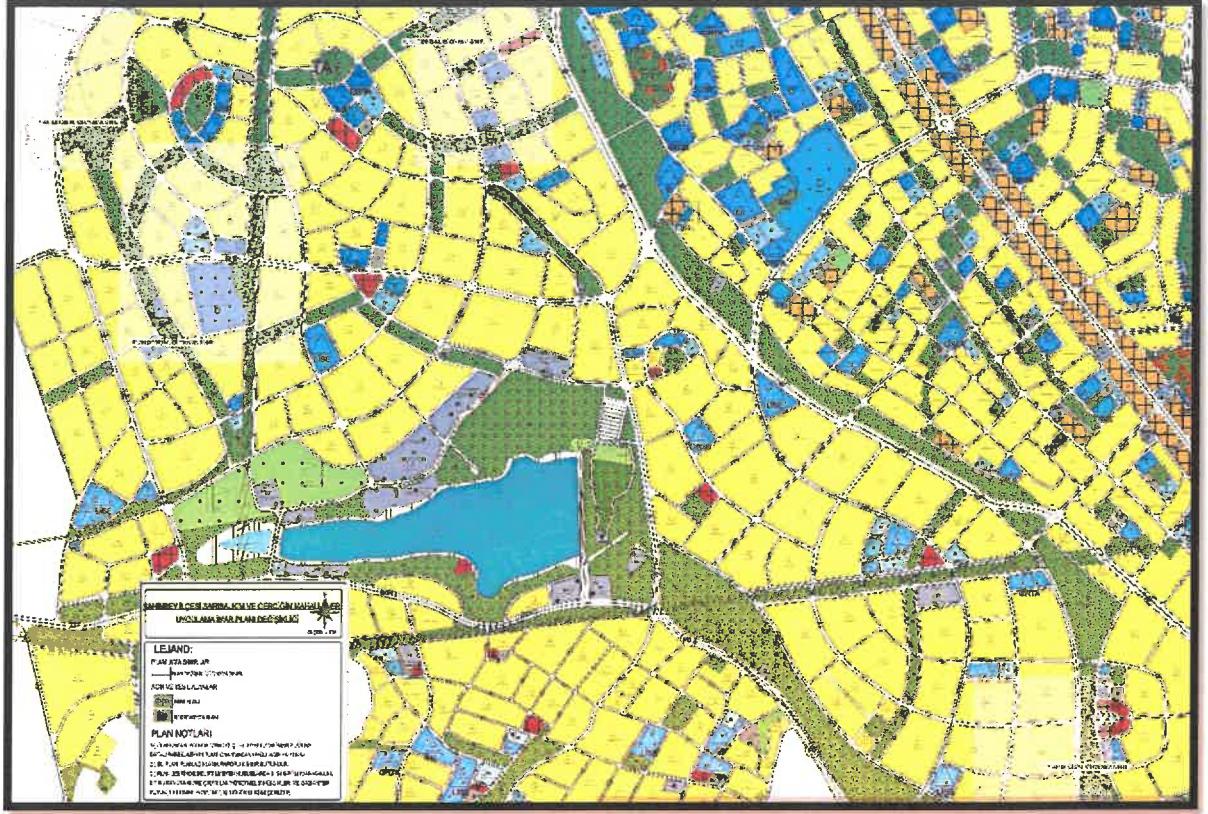
Şekil 3: Şahinbey İlçesi Sarısalkım ve Gerciğin Mahalleleri Planlama Alanı Öneri 1/1000 Ölçekli Uygulama İmar Planı
