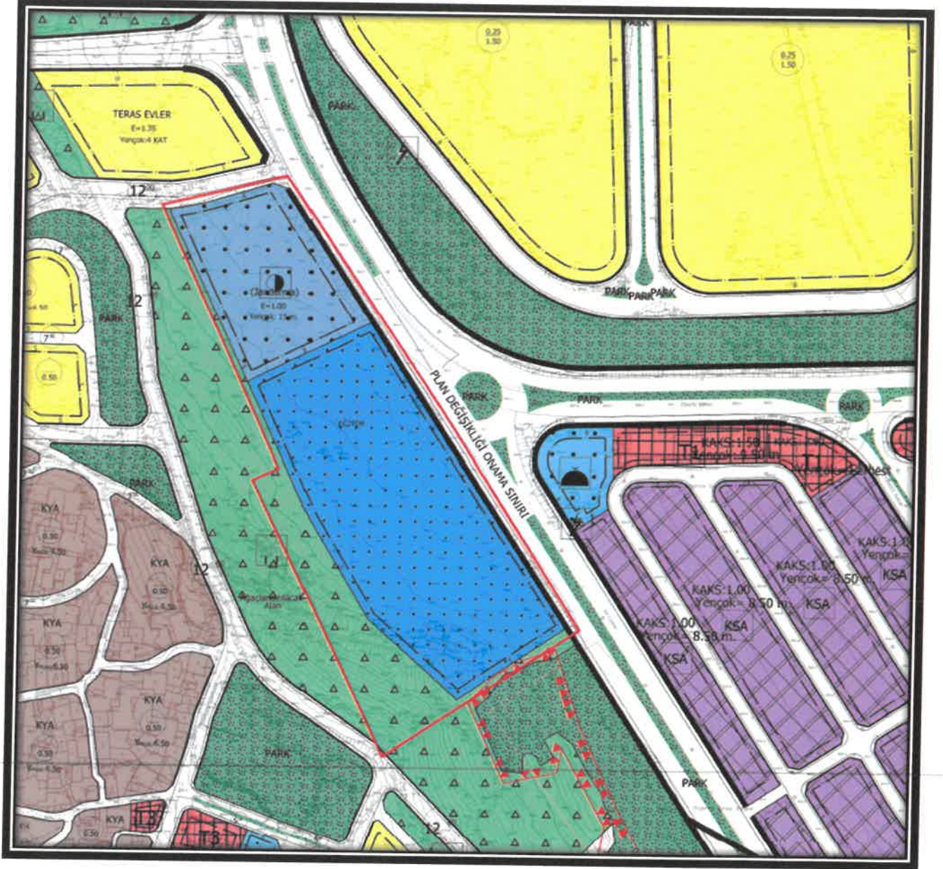
Şekil 3: Planlama Alanı Mevcut 1/1000 Ölçekli Uygulama İmar Planı
