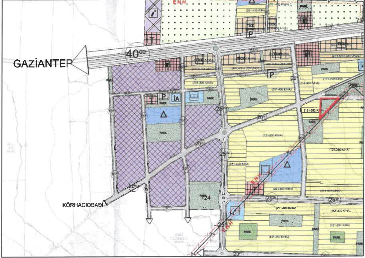
Şekil 2: Planlama Alanının Mevcut 1/5000 Ölçekli Nazım İmar Planındaki Durumu
