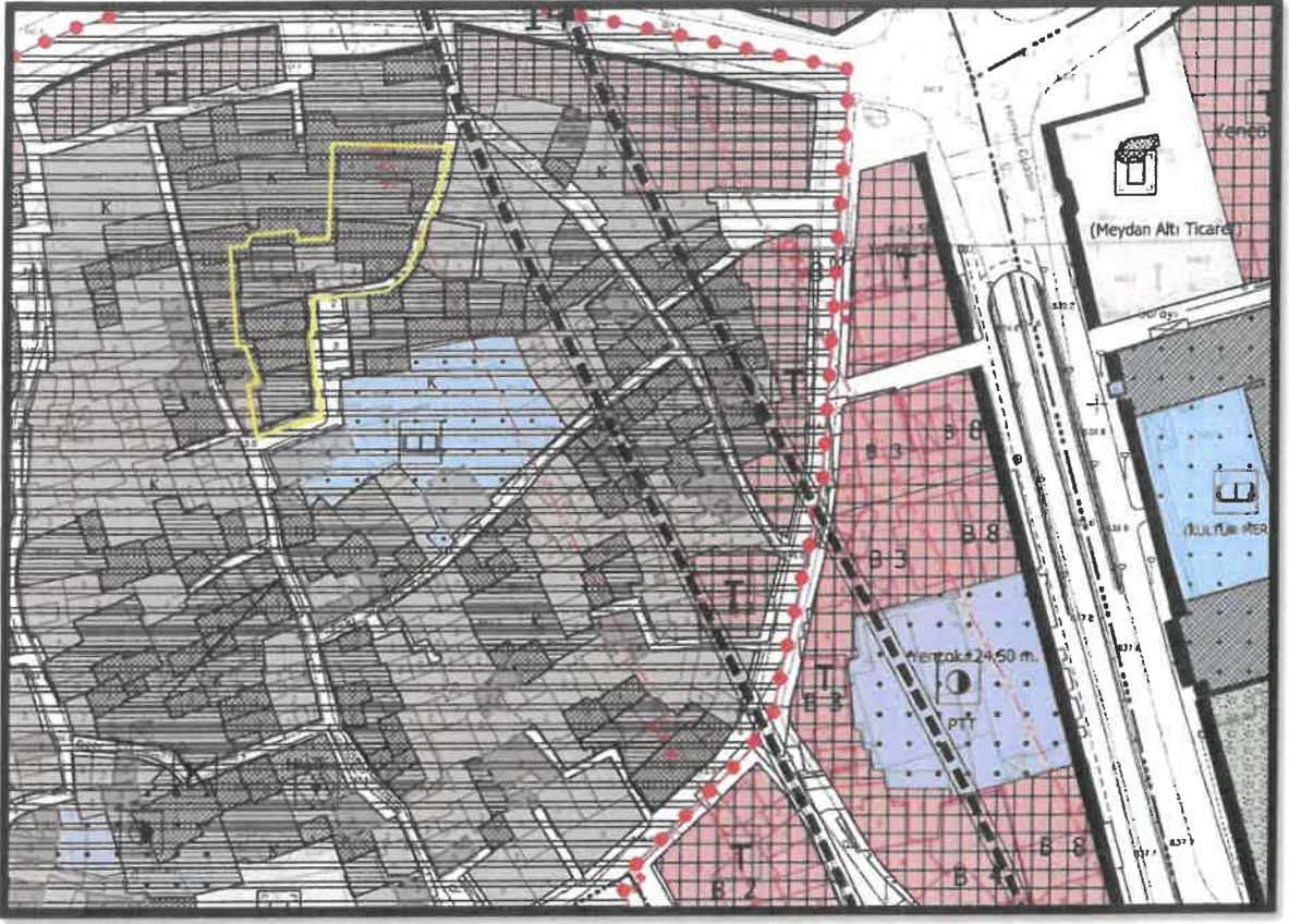
Şekil 2: Planlama Alanı Mevcut 1/1000 Koruma Amaçlı Nazım İmar Planı
