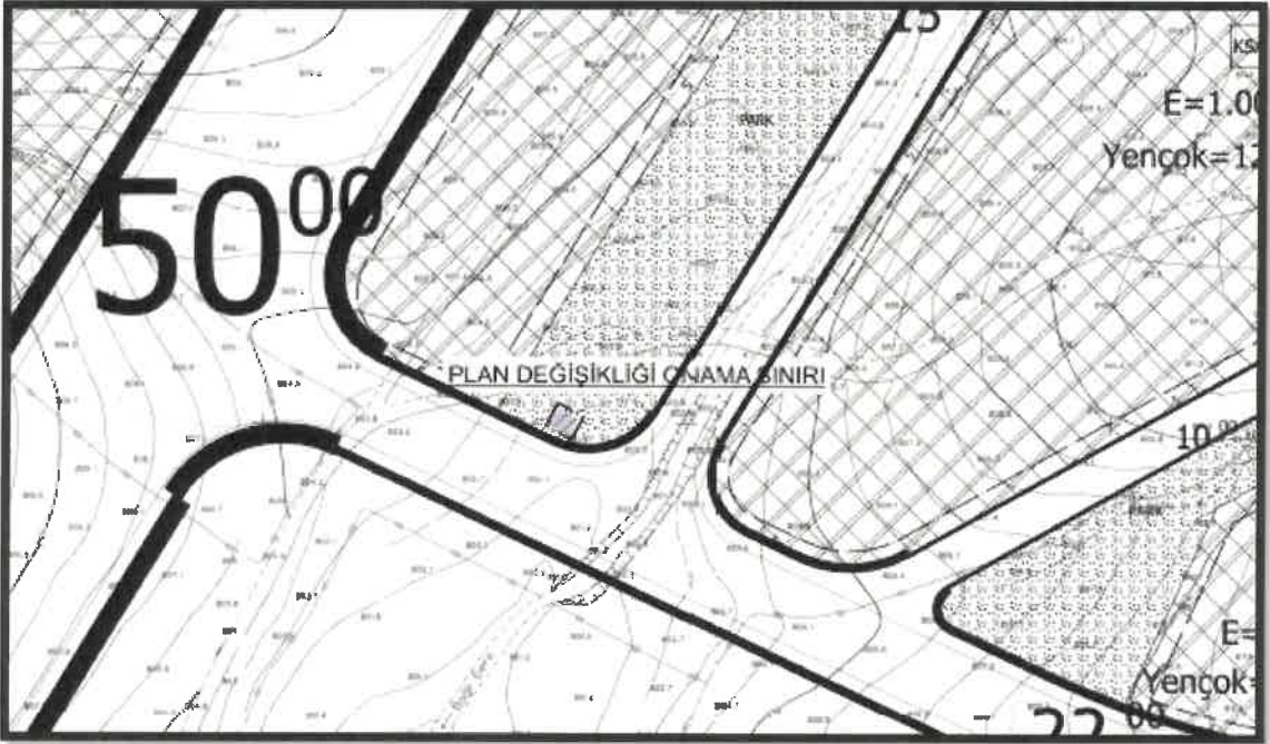
Şekil 3: Önerilen 1/1000 Ölçekli Uygulama İmar Planı
