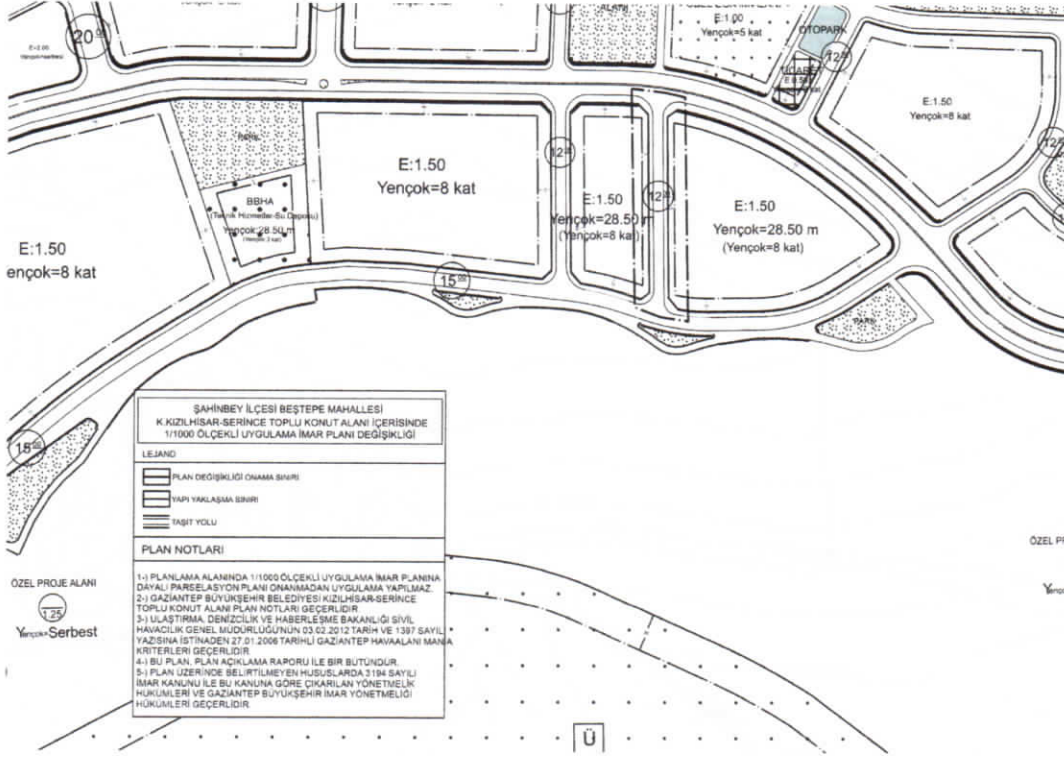
Şekil 3: Planlama Alanı Öneri 1/1000 Ölçekli Uygulama İmar Planı
